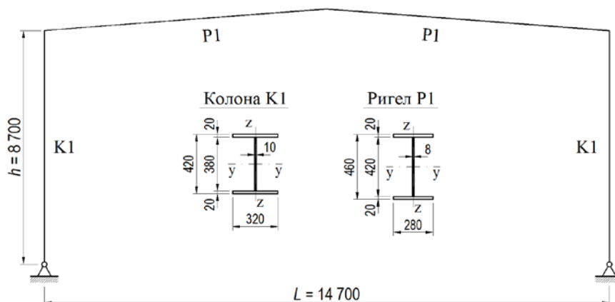
Фиг. 1. Геометрия и статическа схема на типова стоманената рамка, част от сградата в гр. Белово
