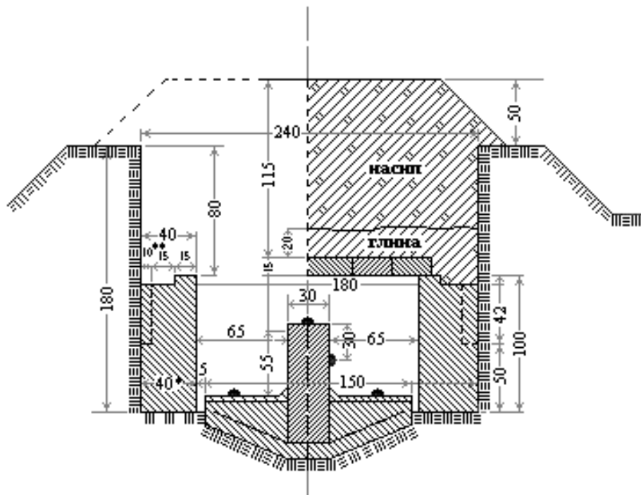
Вертикален разрез а - а
